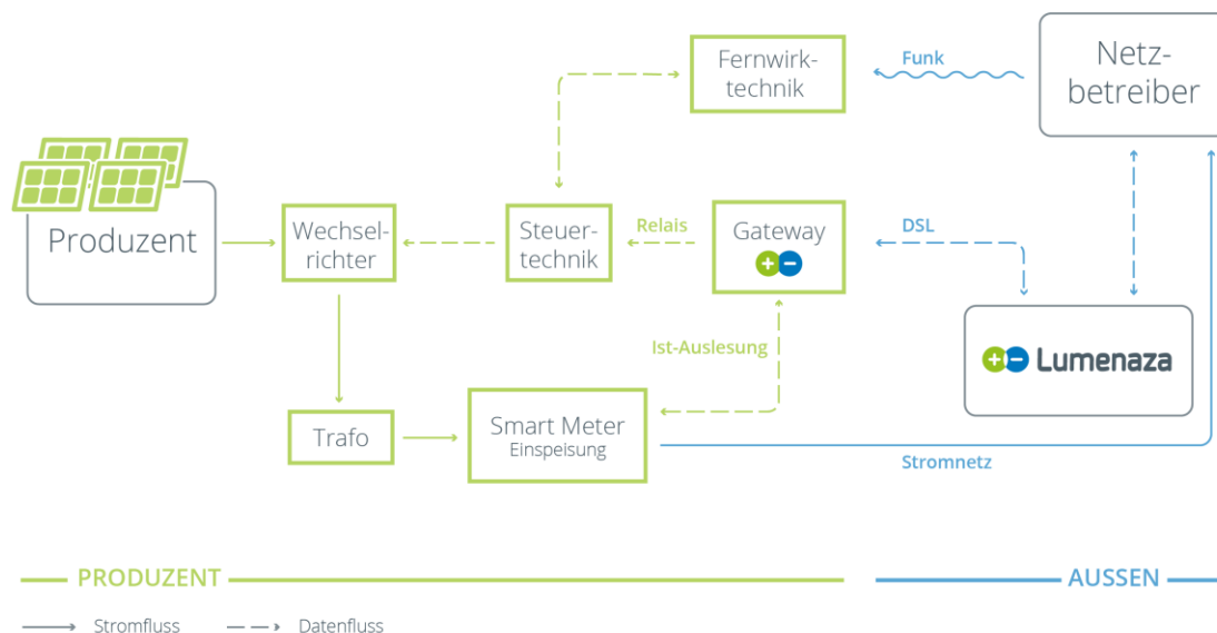
Abbildung 2: Typische Systemkonfiguration in der Direktvermarktung
